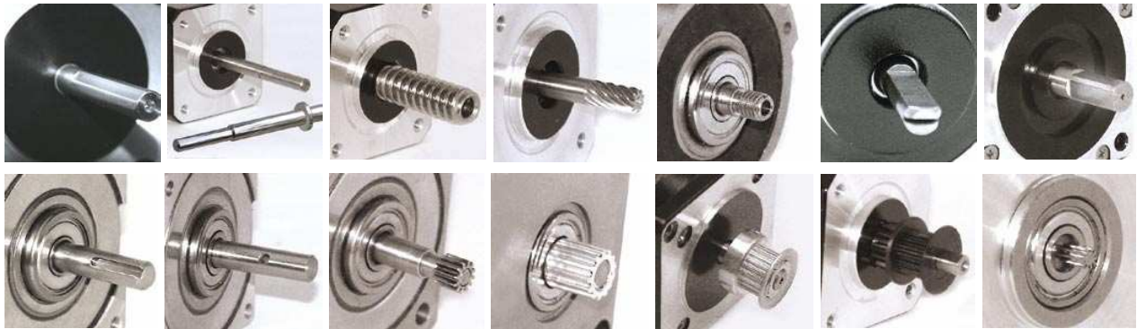
Zahlreiche Wellenvarianten mit Anflachung bis zu verlängerten Zahnrad Passfedern, Schneckenantriebswellen und Durchgangswellen usw.
